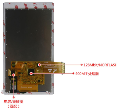
图 1-4 硬件配置图
