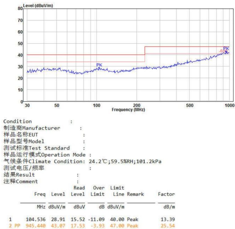
图 7-7 辐射测试垂直方向
